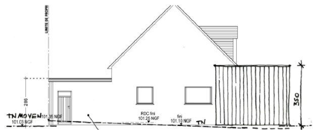
Façade OUEST
