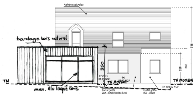
Façade SUD
