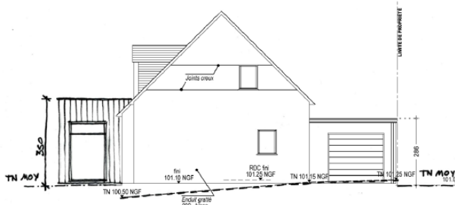
Façade EST
