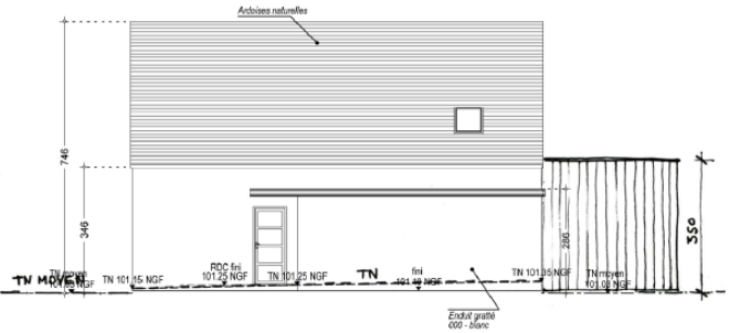
Façade NORD
